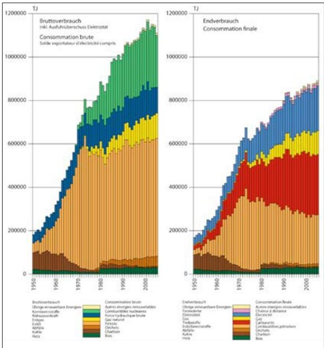
Abb. 2: Energieverbrauch 1950 – 2005 (im TJ)
